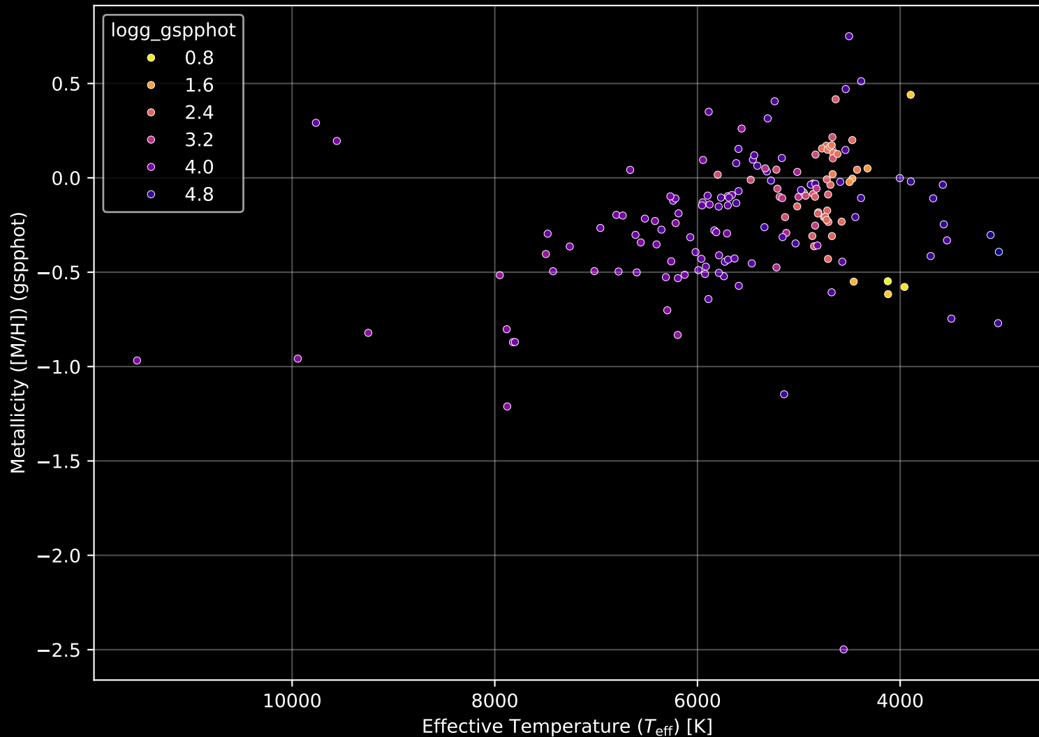
APOGEE DR17 Field: [CVZTILE_095+19_btx] Stellar Population Parameters (n= 169)
